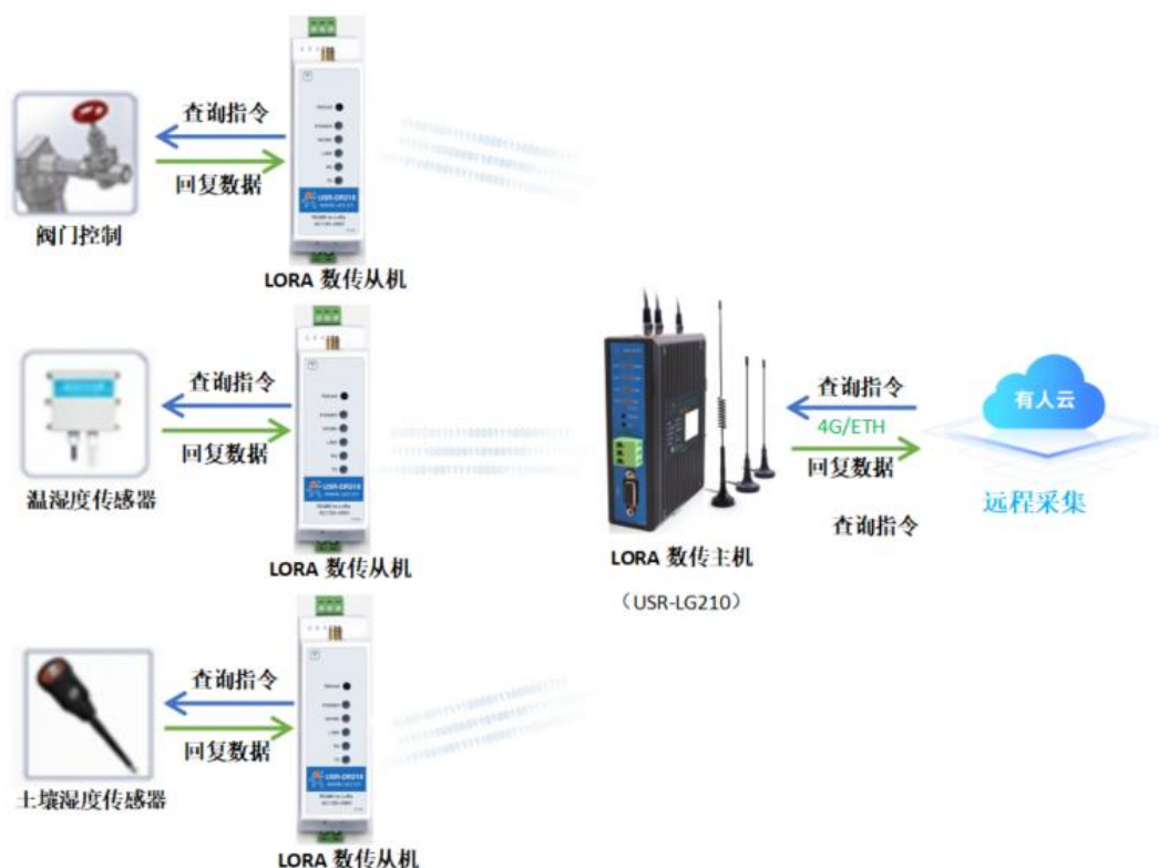
图 3 智慧农业系统示意图
